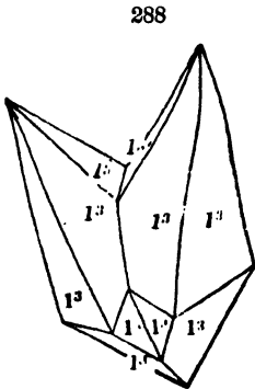
Calcite.
